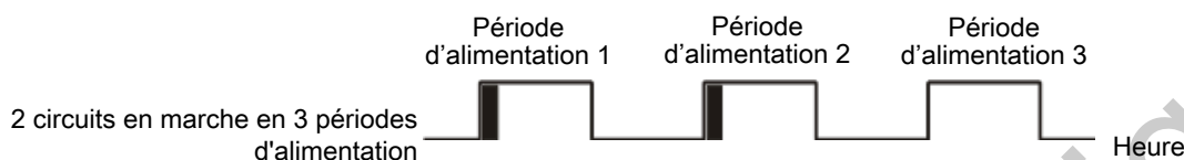
Figure 9: Alimentation par circuit : Exemple 2 : Distribution du nombre de circuits en marche
