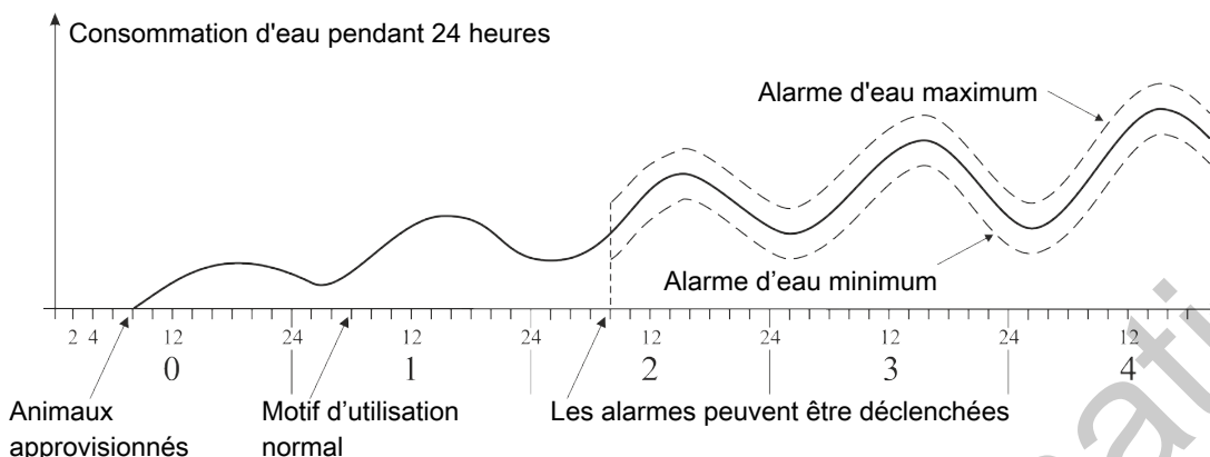
Figure 14: Exemple d'alarme eau minimum et maximum
