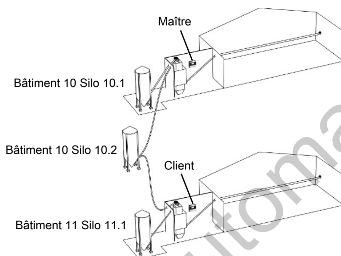
Figure 12: Exemple de silo partagé entre deux bâtiments avec des contrôleurs sur LAN.
