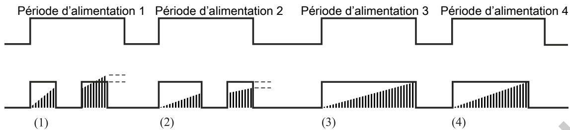
Figure 6: Exemple de correction de consommation d'aliments au cours des périodes.
