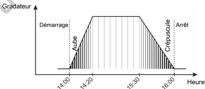
Figure 10: Gradateur normal d'éclairage Aube et crépuscule sont intégrés dans la période d'éclairage.
