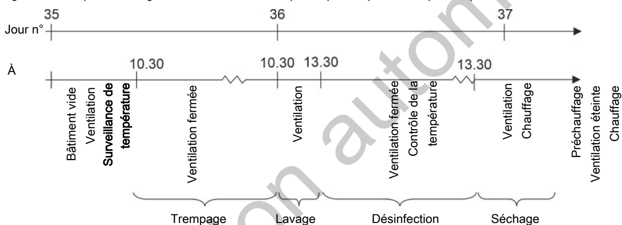
Figure 3: Séquence des fonctions
