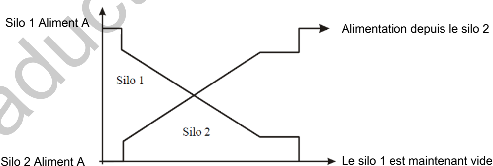
Figure 11: Lorsque le contenu du silo atteint une quantité définie, la transition graduelle vers un autre silo commence.
